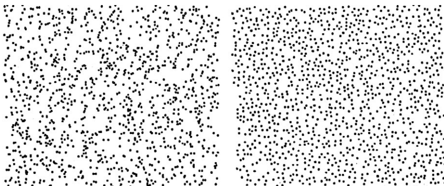
РИС. 5–5. Случайный и неслучайный паттерны
