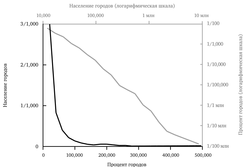
РИС. 5–10. Население городов (степенное распределение), отложенное на линейной и логарифмической шкале
